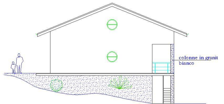
prospetto sud
