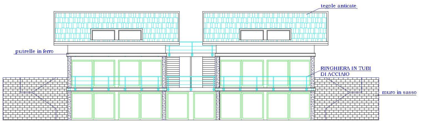
prospetto est
