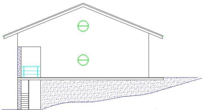
prospetto nord
